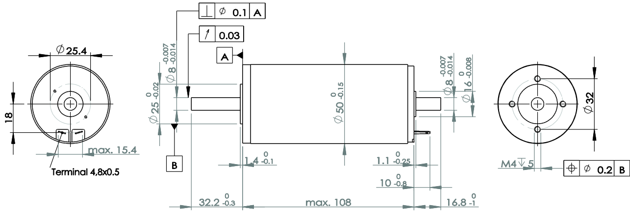
Dimension 尺寸图
